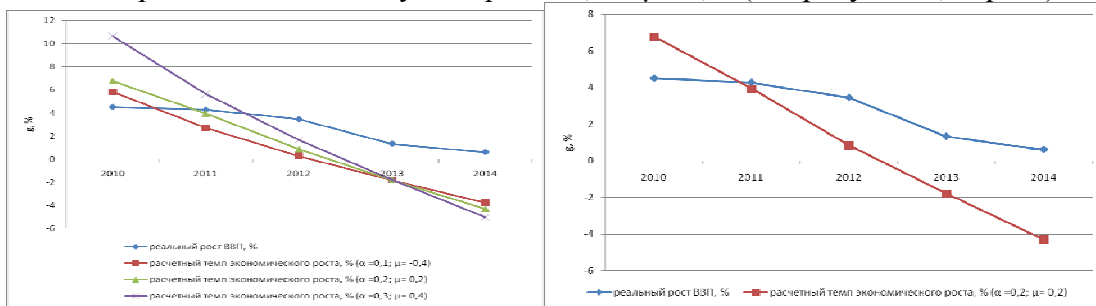
Рисунок 3 - Расчетные и фактическое значение темпа роста в 2010-2014 гг.
